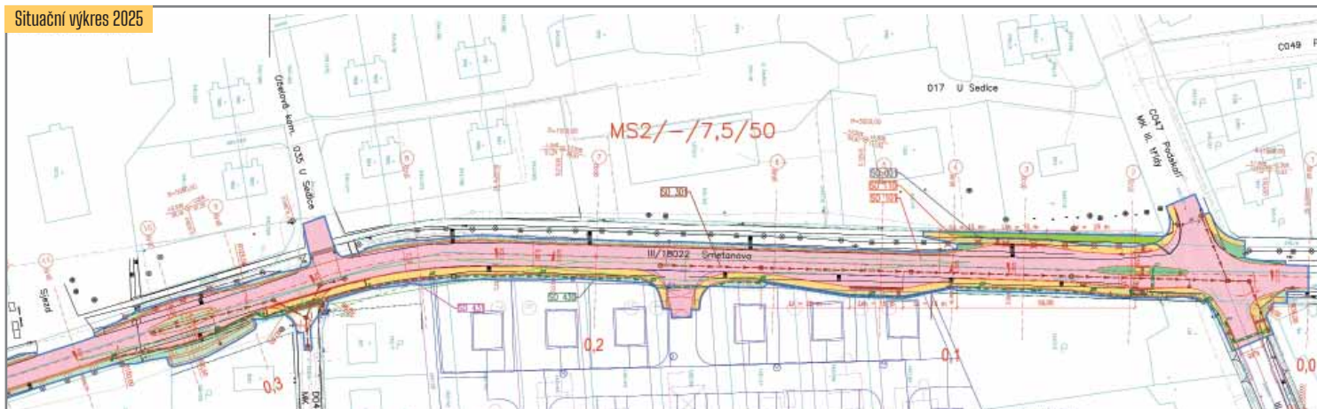
Situační výkres 2025
